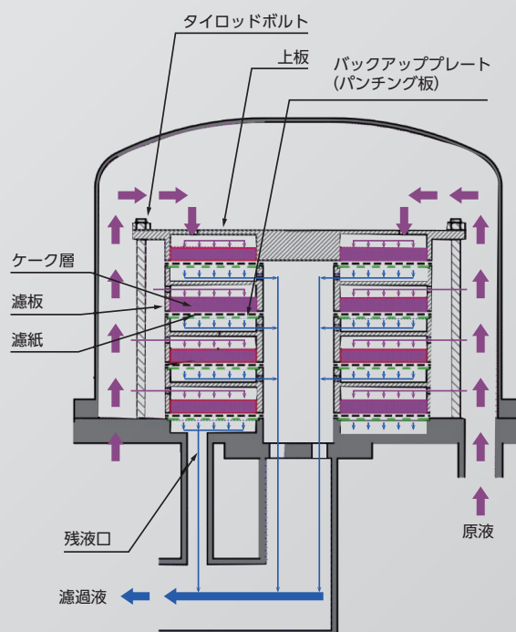
水平濾板濾過機の 断面構造
