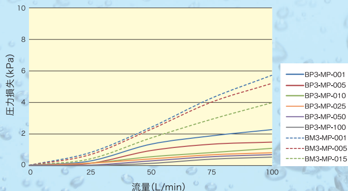
【流量特性】
